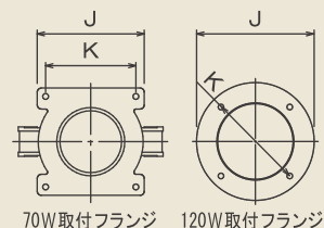
70W取付フランジ 120W取付フランジ
